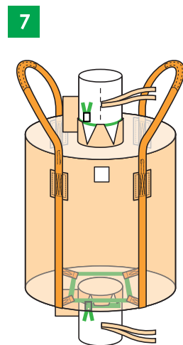
TKW-006 (投入口・排出口付)
